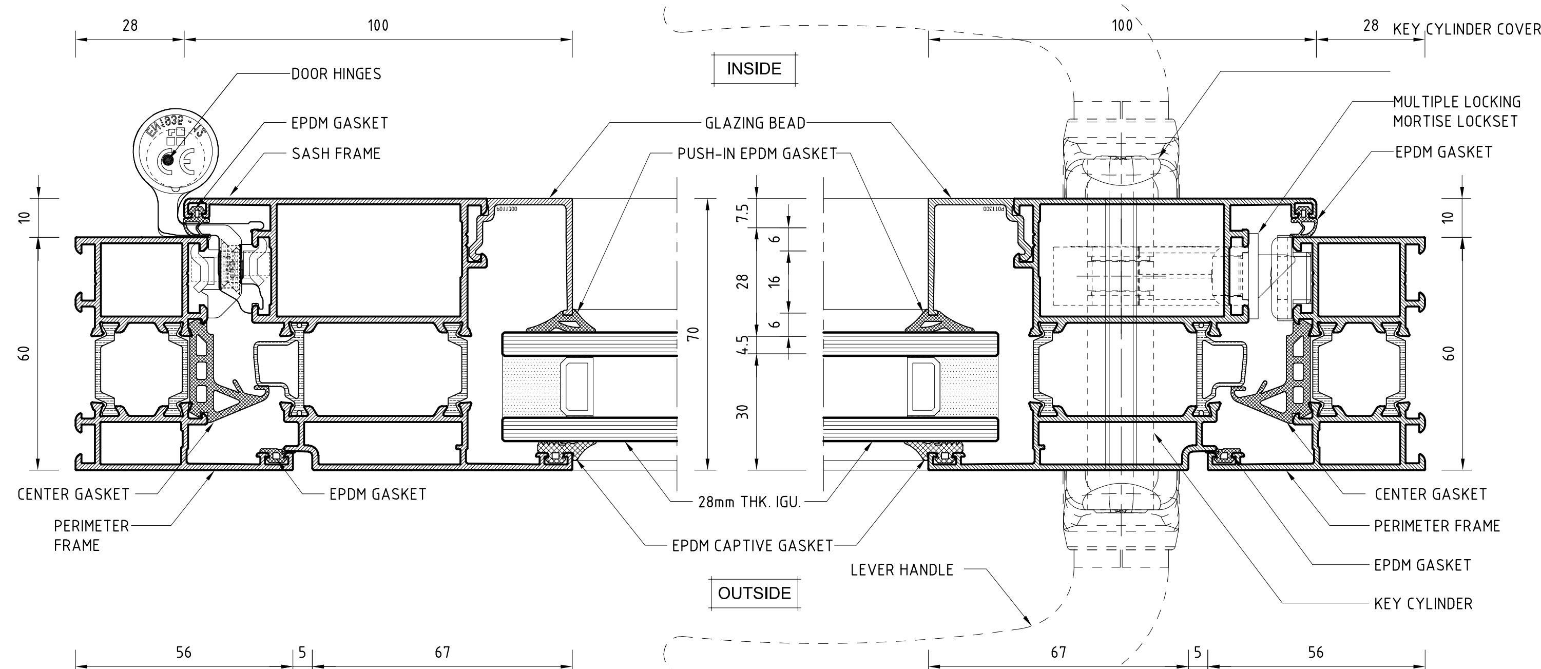
JAMB DETAIL
